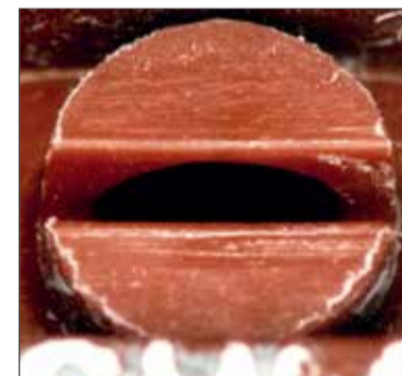
После 200 часов работы с кремниевой кислотой (размер капель 300 мкм, давление 2 бар) отверстие щелевой форсунки стало на 20 - 30 % шире.
